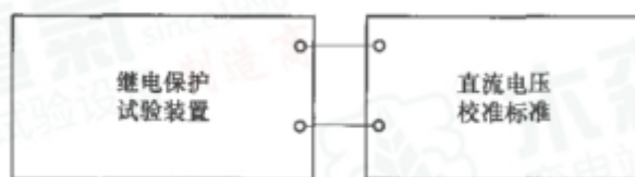
图9 直流电压校准接线示意图
