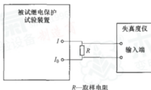
图 3 交流电流总谐波畸变率测量接线图
