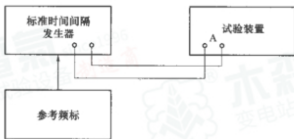
图 14 时间测量检验试验线路图
