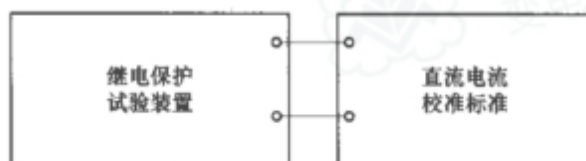
图 7 直流电流校准接线示意图
