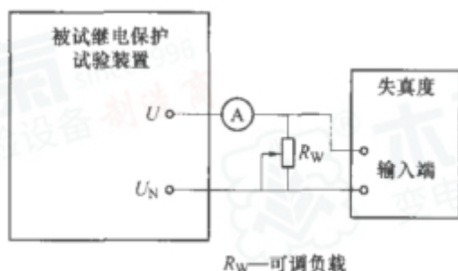
图 6 交流电压总谐波畸变率测量接线图
