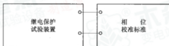
图 11 相位校准接线示意图
