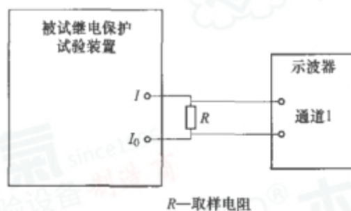
图 2 交流电流响应速度测量接线图
