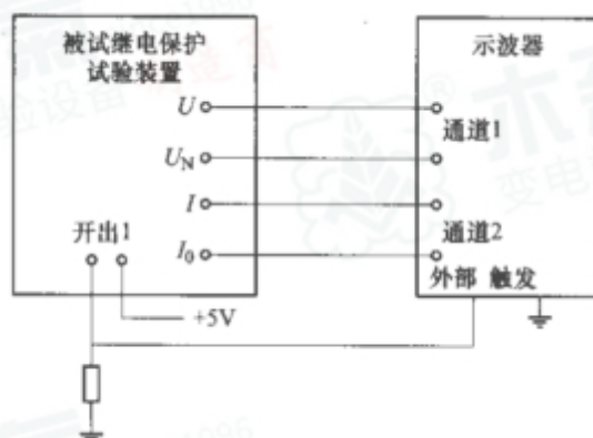
图 12 合闸相位角试验接线图
