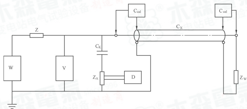
图 3 电桥线路
