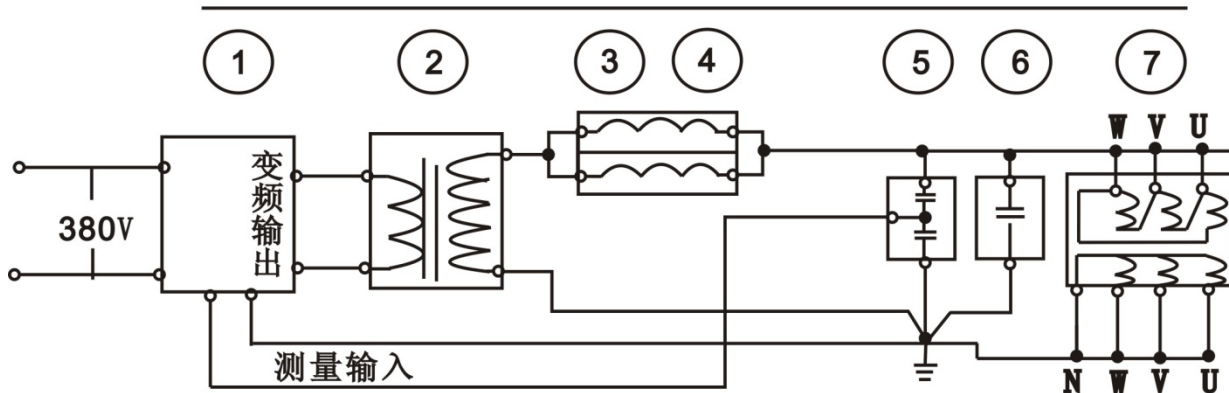
变压器耐压试验接线图
