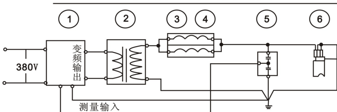
电缆耐压试验接线图
