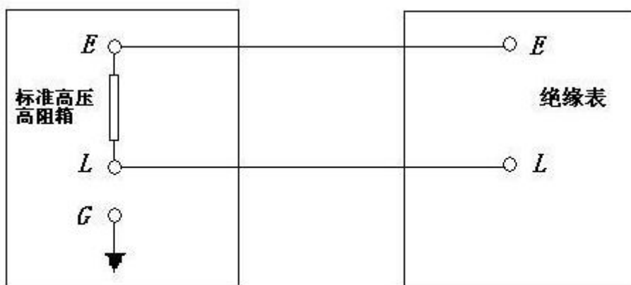
图 1 检测基本误差接线图
