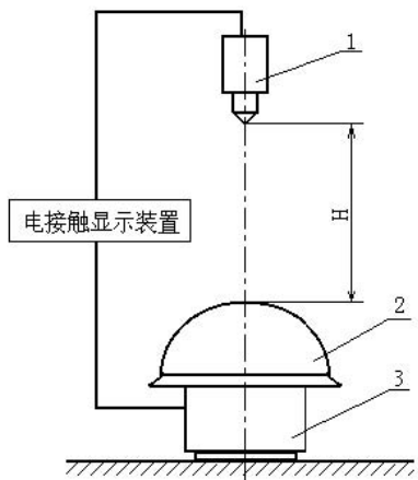
图10 耐穿刺性能试验示意图
