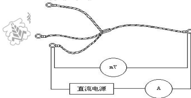
图1 携带型短路接地线成组直流电阻试验
