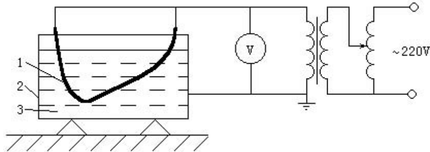
图2 连接导线绝缘强度试验
