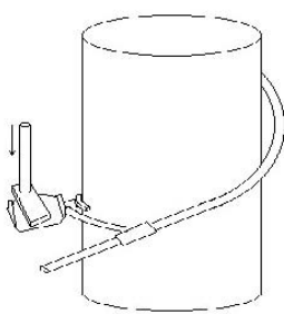
图11 脚扣试验示意图
